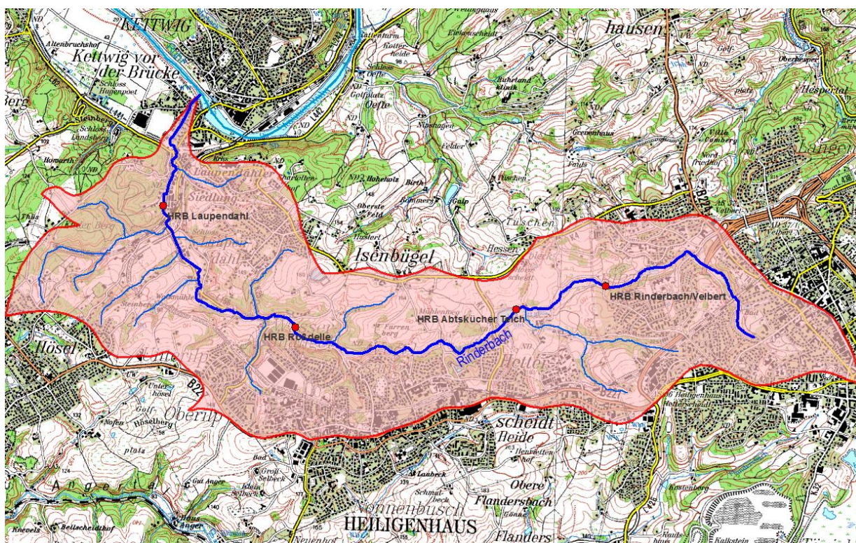
Abbildung 2-2 HRB im Einzugsgebiet des Rinderbachs
