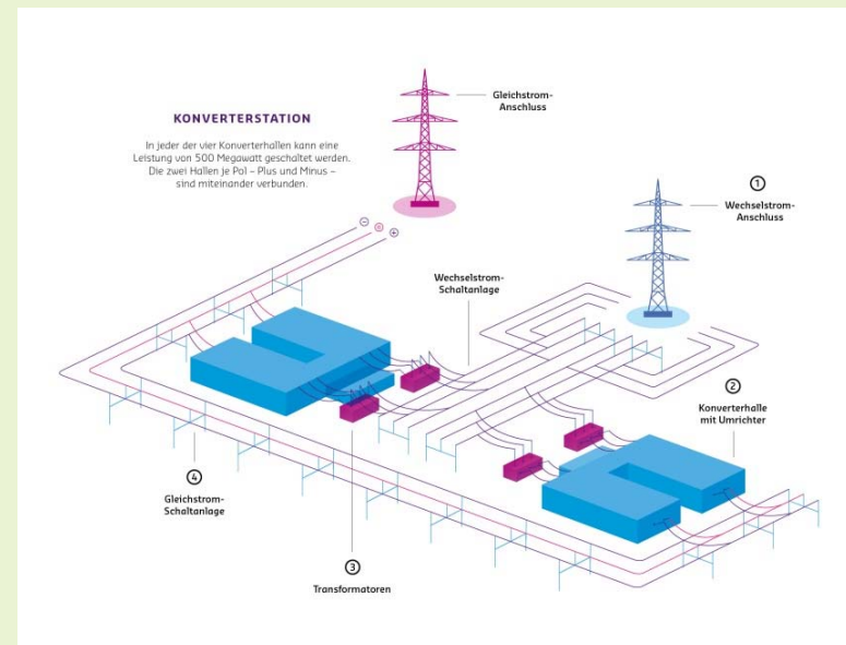
Schematische Darstellung eines Konverters (Quelle Firma Amprion)
