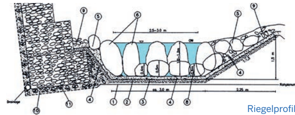
Riegelprofil
