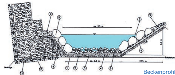
Beckenprofil
